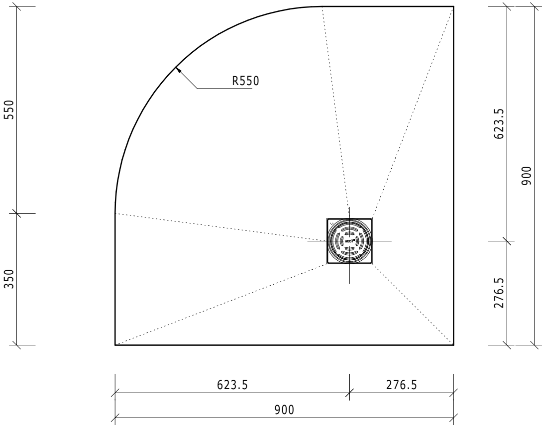
Draufsicht
