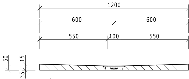
Schnitt A-A
