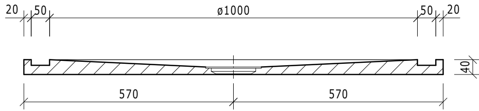
Schnitt
