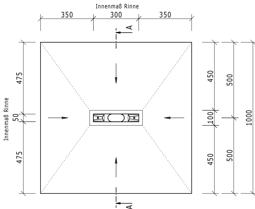
Draufsicht
